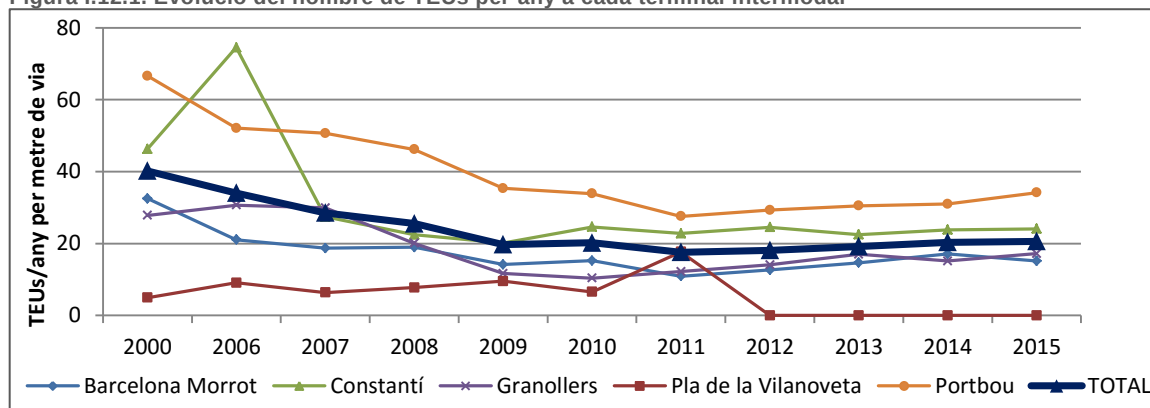
Figura I.12.1. Evolució del nombre de TEUs per any a cada terminal intermodal
