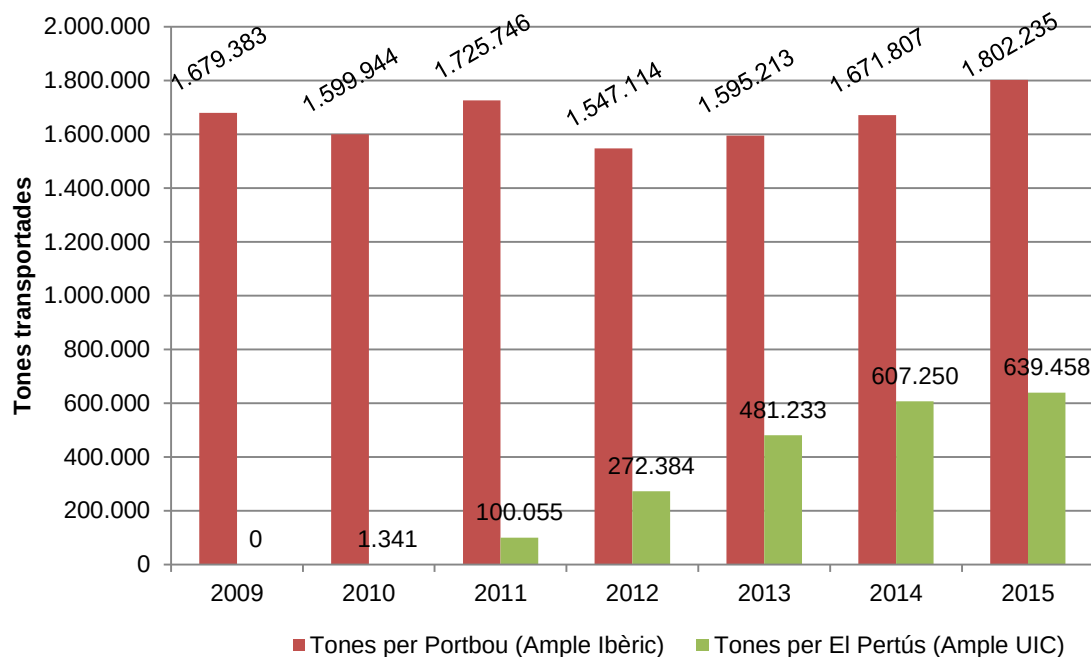
Figura III.18.1. Tràfic ferroviari transpirinenc expressat en tones transportades
